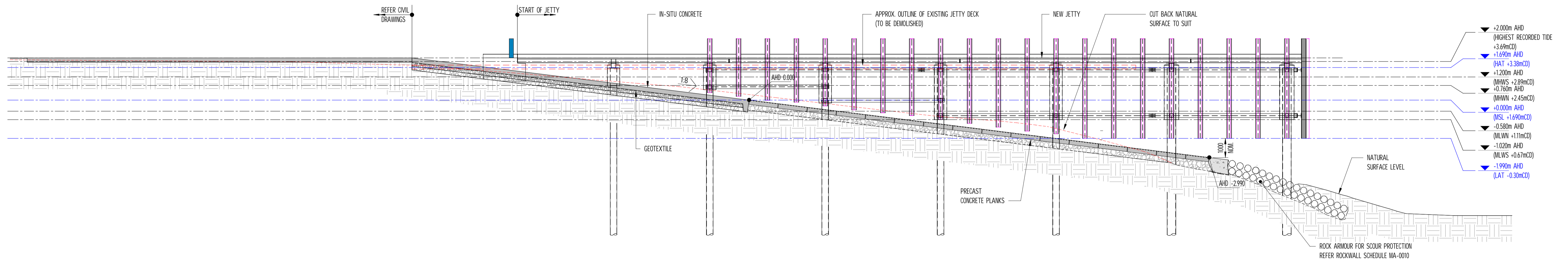
SECTION SCALE 1 : 100
